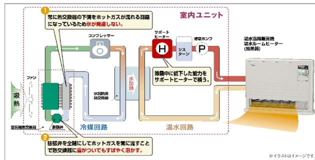
ヒートポンプ式温水温風暖房システム
